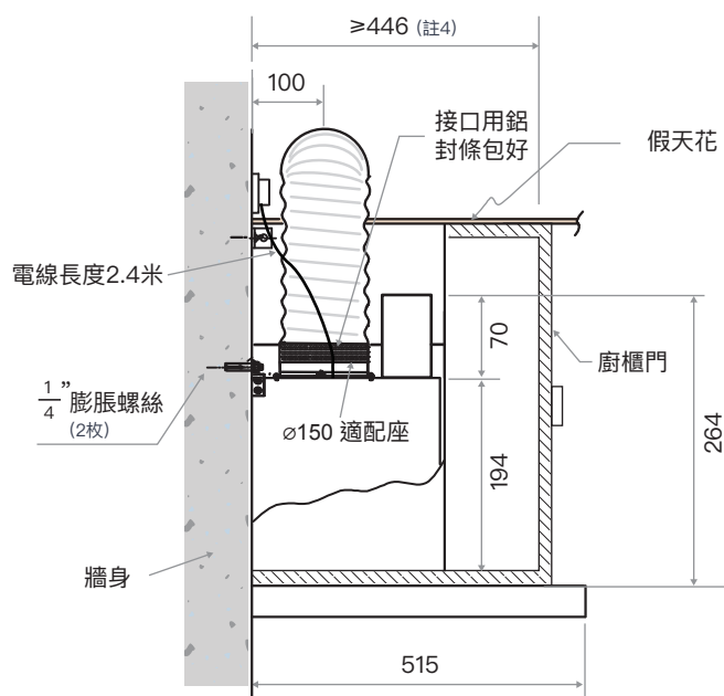
側視圖
