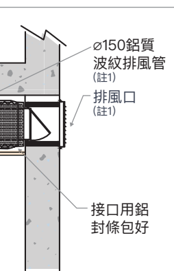
排風口在牆身
