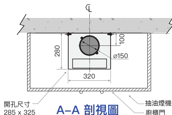
排風口在牆身
