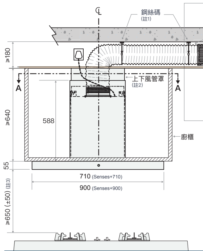
正視圖
