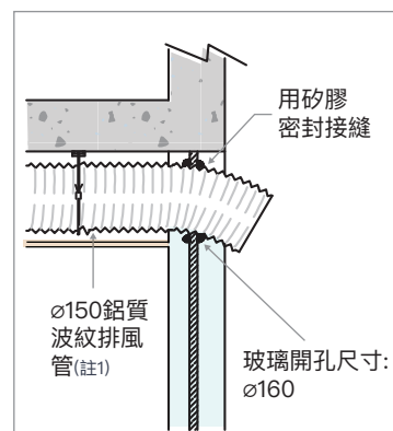
排風口在玻璃
